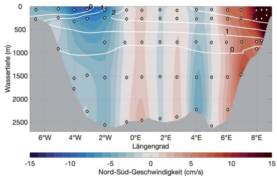
Abbildung 5. Mittleres Geschwindigkeitsfeld durch die Framstraße (in Abb. 3 bei 79°N) zwischen Grönland (links) und Spitzbergen (rechts). Die schwarzen Rauten markieren die Positionen der verankerten Strömungsmesser (Exkurs 1). Das nach Norden gerichtete Strömungsband (rot) auf der rechten Seite ist der Westspitzbergenstrom, das süd-wärtige Band links der Ostgrönlandstrom. Die weißen durchgezogenen Konturen stellen Linien gleicher Temperatur dar. Man kann erkennen, dass auch der nach Süden gerichtete Strom warmes Atlantikwasser enthält.
