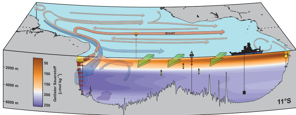
Abbildung 11. Schematische Darstellung der Zirkulation im tropischen Atlantik, des Beobachtungssystems bei 11°S und der Langzeitverankerung am Äquator bei 23°W. Die rötlichen Pfeile repräsentieren die Warmwasserströmungen im oberen Ozean einschließlich des Nordbrasilianischen Unterstroms (NBUC) und seinem Abzweig zum Äquatorialen Unterstrom (EUC). Blaue Pfeile stellen die Zirkulation des Tiefenwassers aus dem Nordatlantik, violette Pfeile die Ausbreitung des antarktischen Bodenwassers und grüne Pfeile den windgetriebenen Transport bei 11°S dar. Der Vordergrund zeigt die Sauerstoffverteilung entlang von 11°S; hier fallen der Westliche Randstrom und Umgebung durch einen hohen Sauerstoffgehalt auf. Ursache dafür ist, dass das Tiefenwasser im Randstrom auf dem schnellsten Weg bis 11°S geströmt ist und der Sauerstoff deshalb noch nicht so stark verbraucht wurde wie bei älterem Tiefenwasser.
